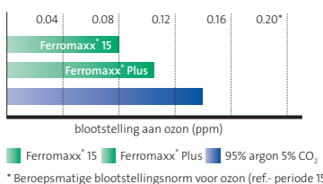
Gemiddelde blootstelling aan ozon bij handmatig MAG-lassen van koolstofstalen platen bij sproeibooglassen
